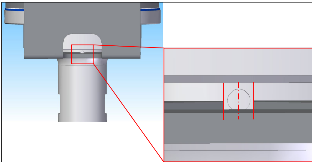
Fig. 8.3.1 (d) J4-axis zero degree position
