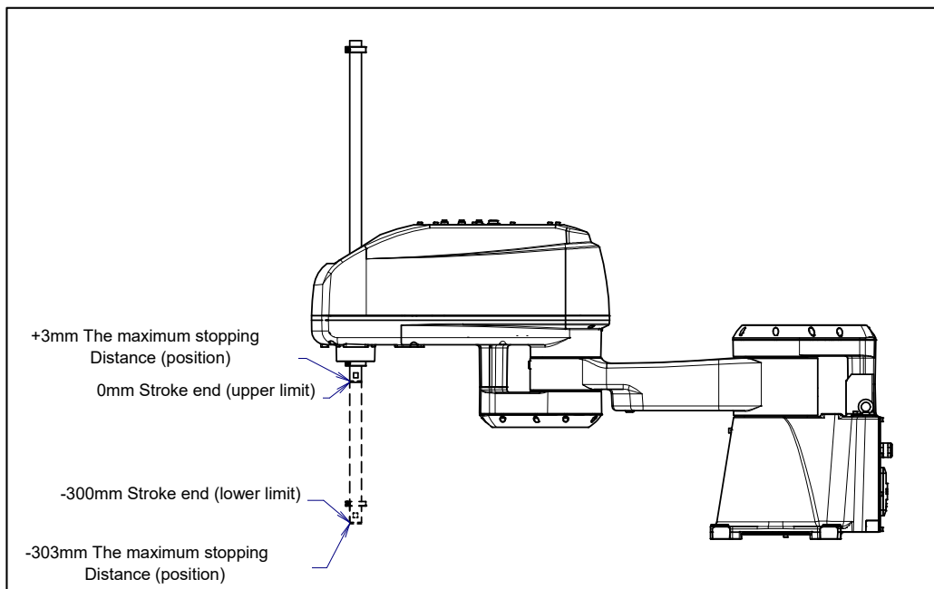
Fig. 3.3 (d) J3-axis motion limit (300mm stroke)
