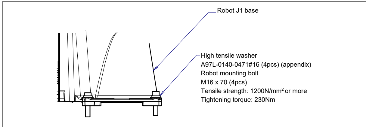
Fig. 1.2.1 (a) Actual Installation Example
